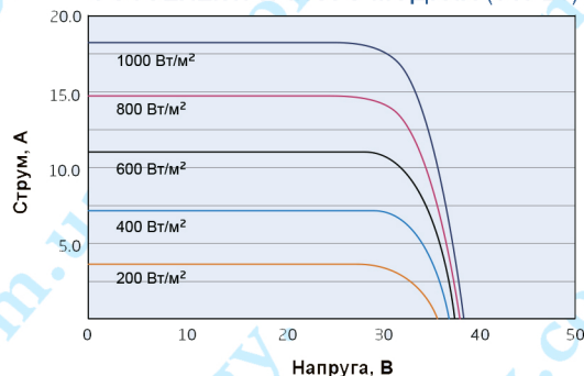
ВОЛЬТ-АМПЕРНІ ХАРАКТЕРИСТИКИ ФОТОЕЛЕКТРИЧНОГО МОДУЛЯ (545 Вт)
