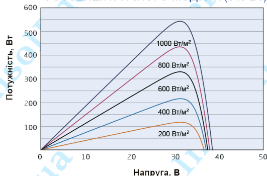
КРИВІ ПОТУЖНІСТЬ-НАПРУГА ФОТОЕЛЕКТРИЧНОГО МОДУЛЯ (545 Вт)
